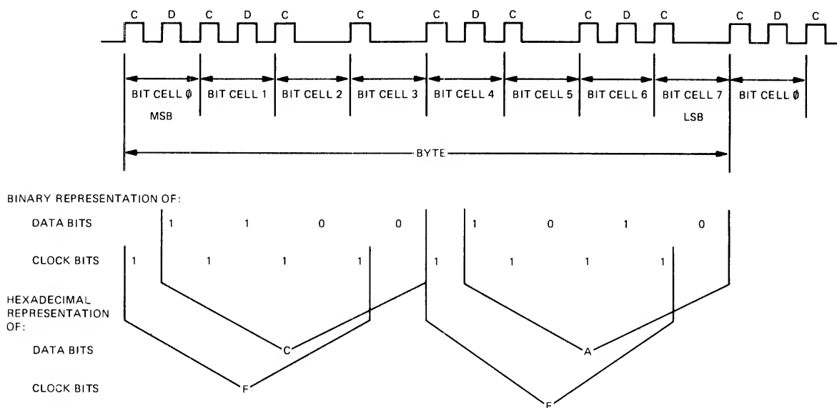
FIGURE 19. BYTE
